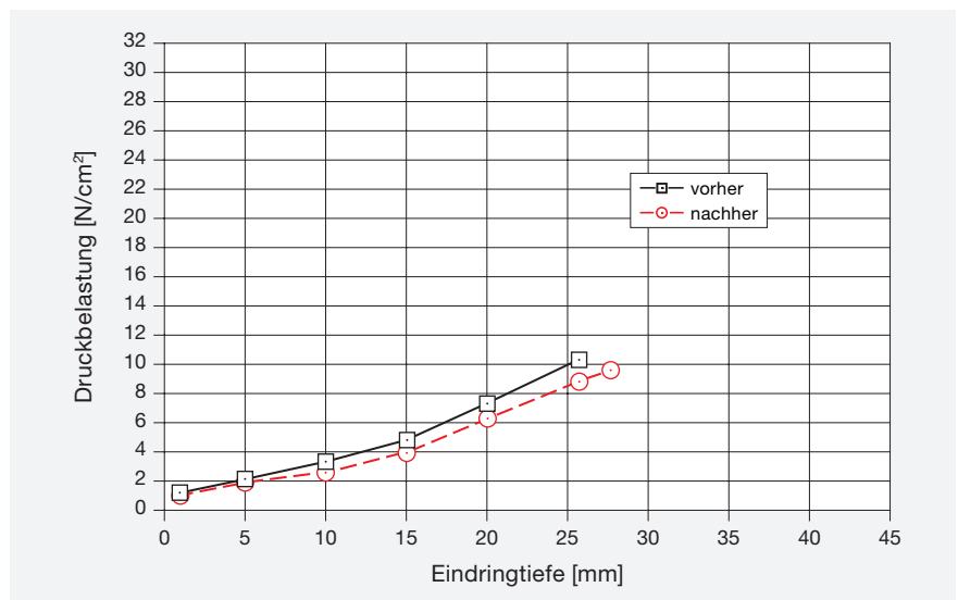
Bild 3: Verformbarkeit, Eindringtiefe der Kalotte ( r = 120 \text{ mm} ) in Abhängigkeit vom Auflagedruck
